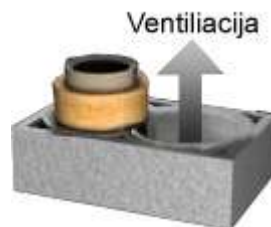
Ø 160 + 0 dvigubas modulis, šamoto vidinis diametras 160 mm, laisva anga paliekama ventiliacijai
